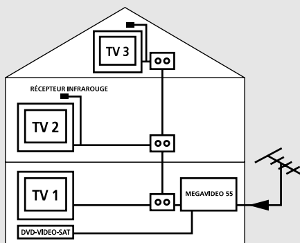
récepteur infrarouge
