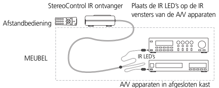
Fig 2 Afstandsbediening
