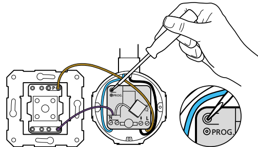
Figuur 10. Activeren en opheffen van de programmeermodus.
